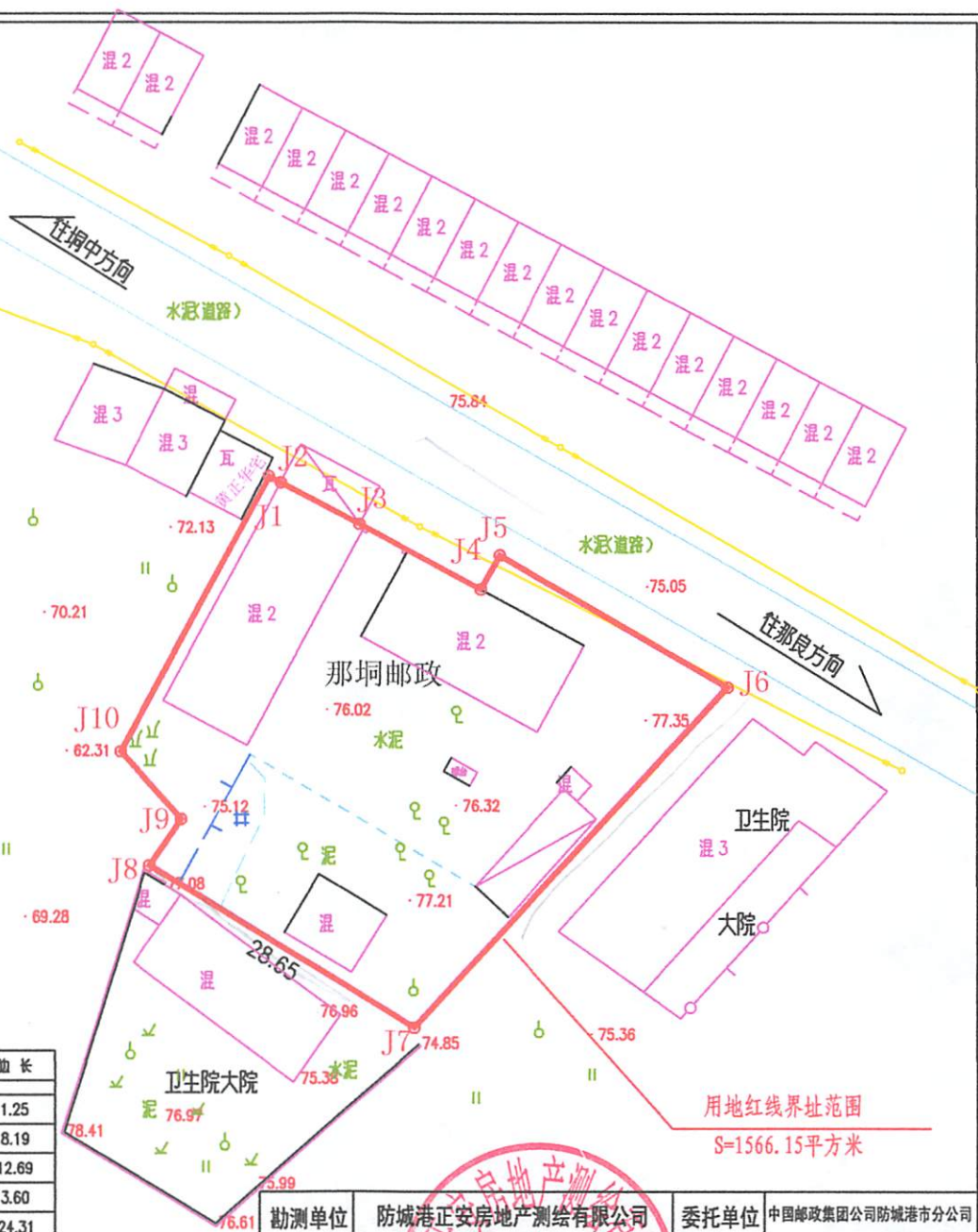
界址点坐标表
